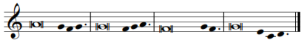
Psalm 93
